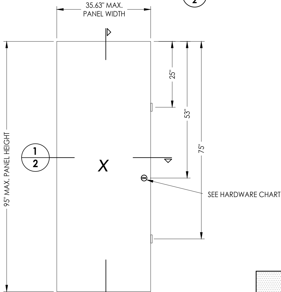
2 2 DOOR PANEL MastergGrain
