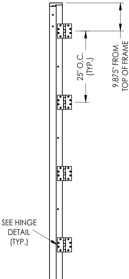
HINGE JAMB
